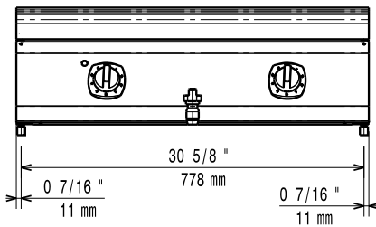
Front aanzicht
